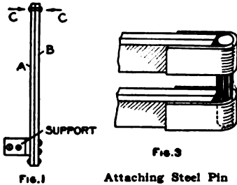
Simple Thermostat
