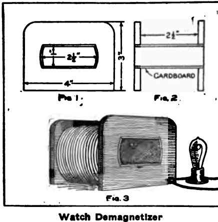
Watch Demagnetizer
