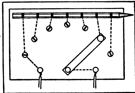
Simple Rheostat
